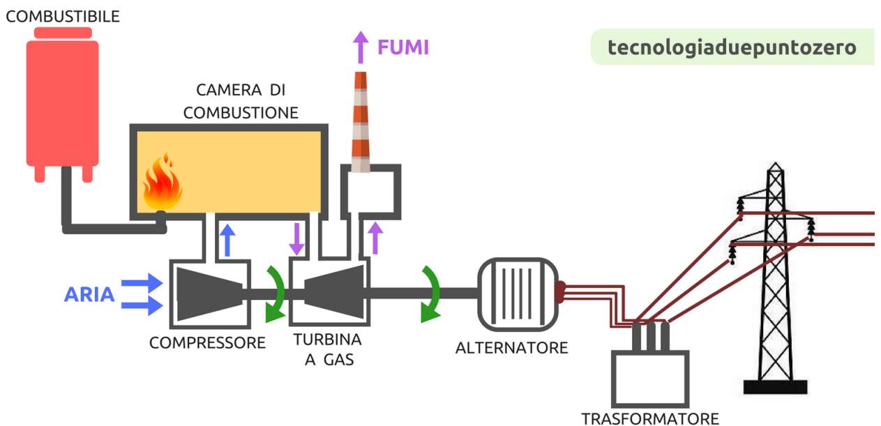
Schema di funzionamento di una CENTRALE TERMOELETTRICA A TURBOGAS
